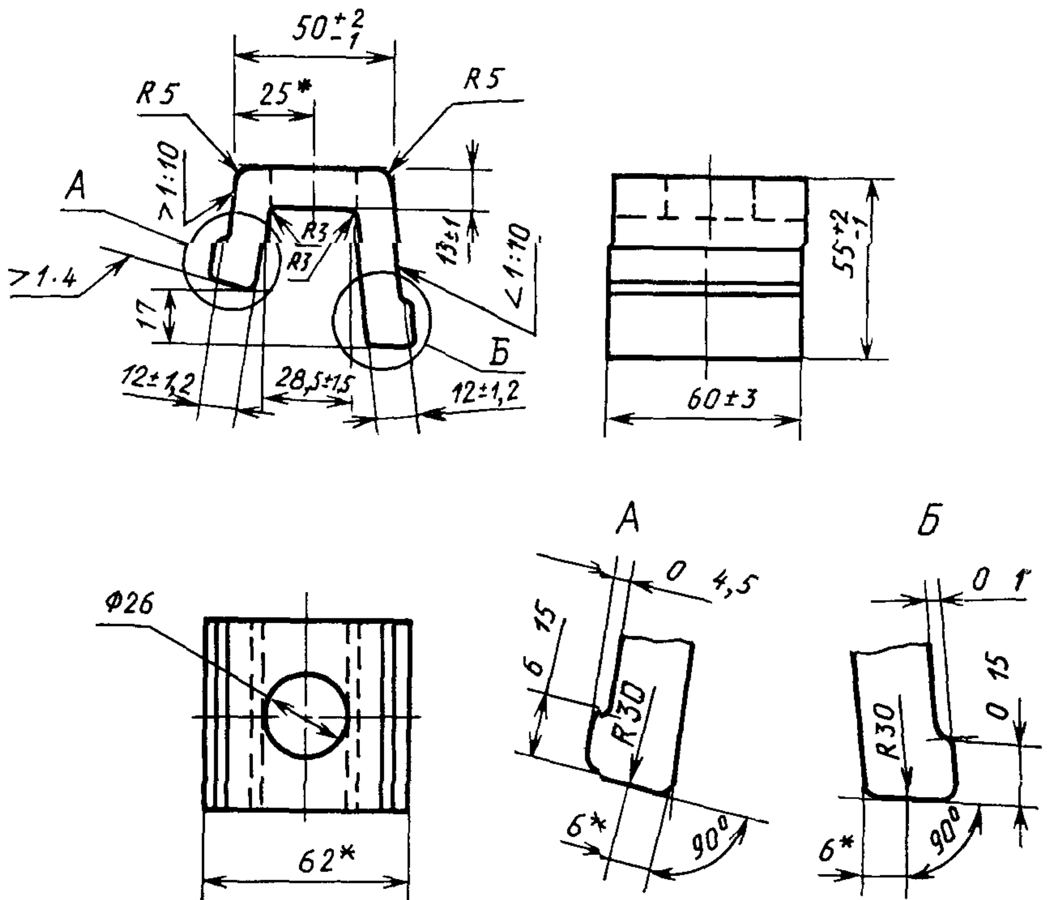
Клемма ПК
