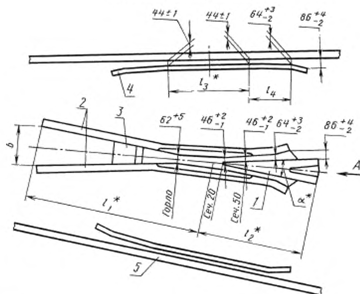
Крестовина с контрельсами
