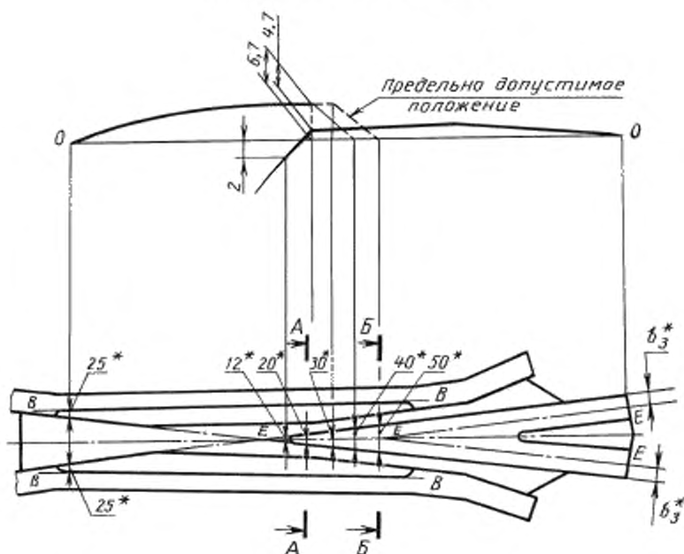
Продольный профиль крестовины
